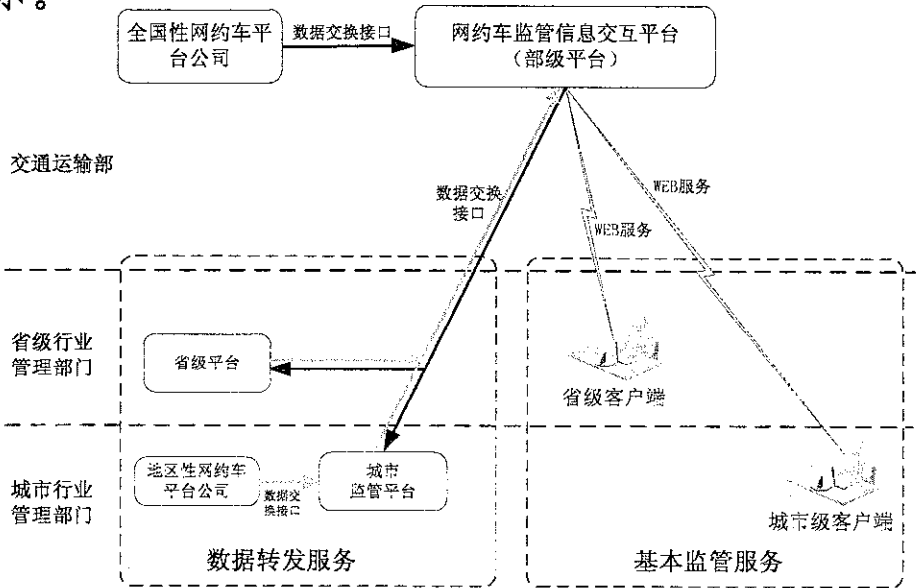
图 5—1 总体架构图
